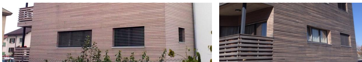
Façade en mélèze prégrisé, à la construction et après 8 ans
